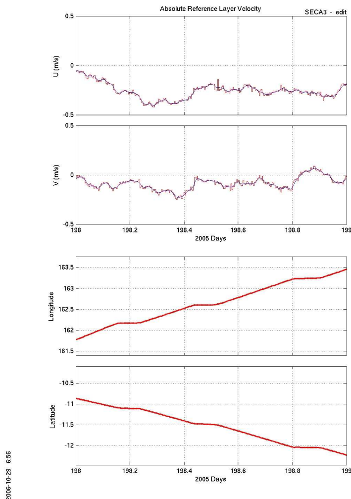
Figure 19 : Exemple de courant dans la couche de référence 38-102m, après nettoyage des profils individuels (« édition ») et lissage. Les 2 derniers graphiques montrent la navigation.
